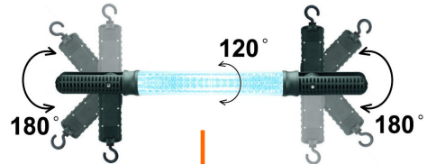
本体チューブは最大120°回転します。
